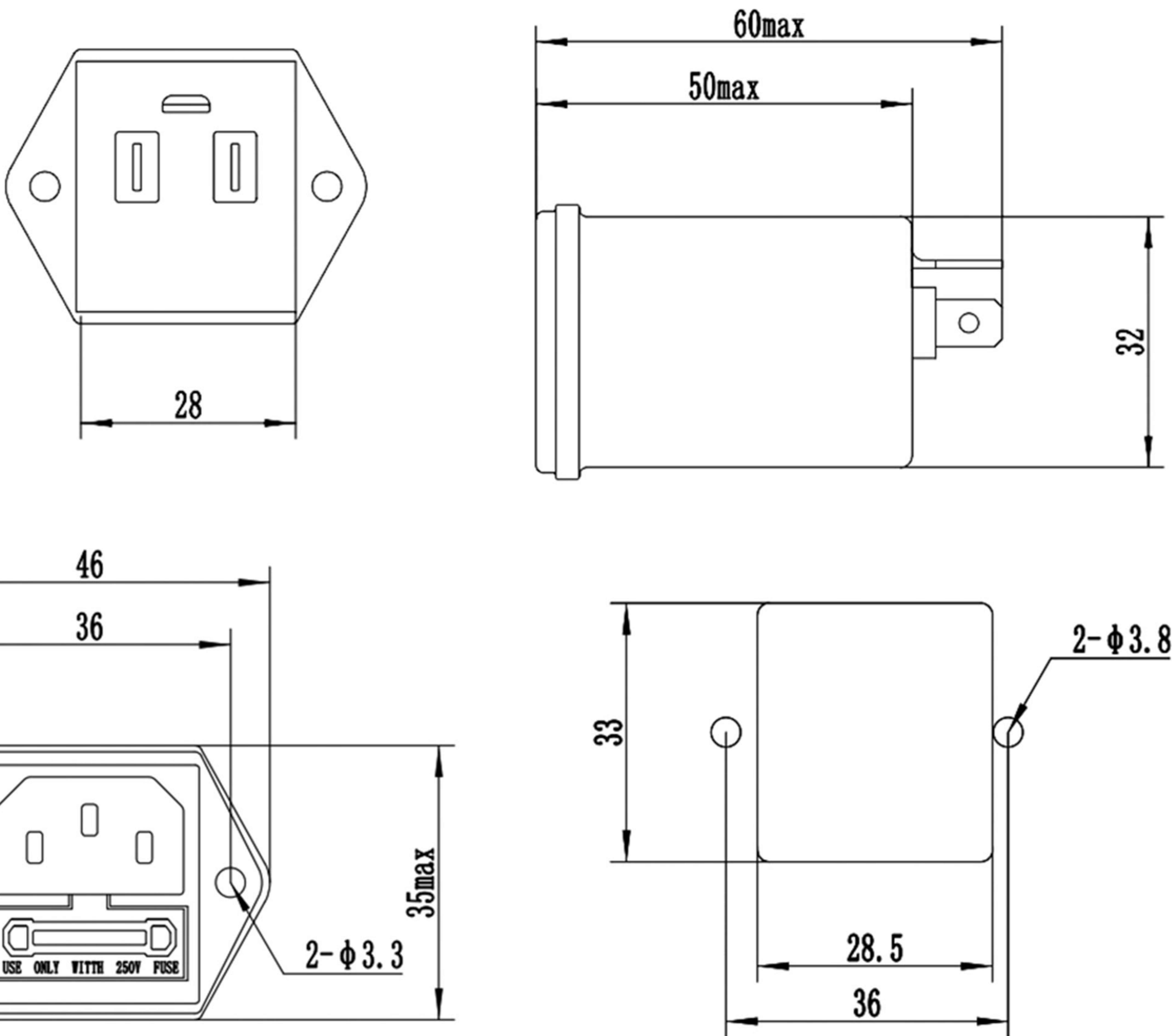
安装尺寸示意图
